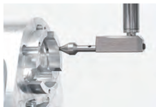
Anwendungsbeispiel
