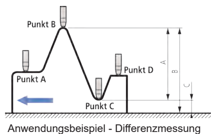
Anwendungsbeispiel - Differenzmessung
